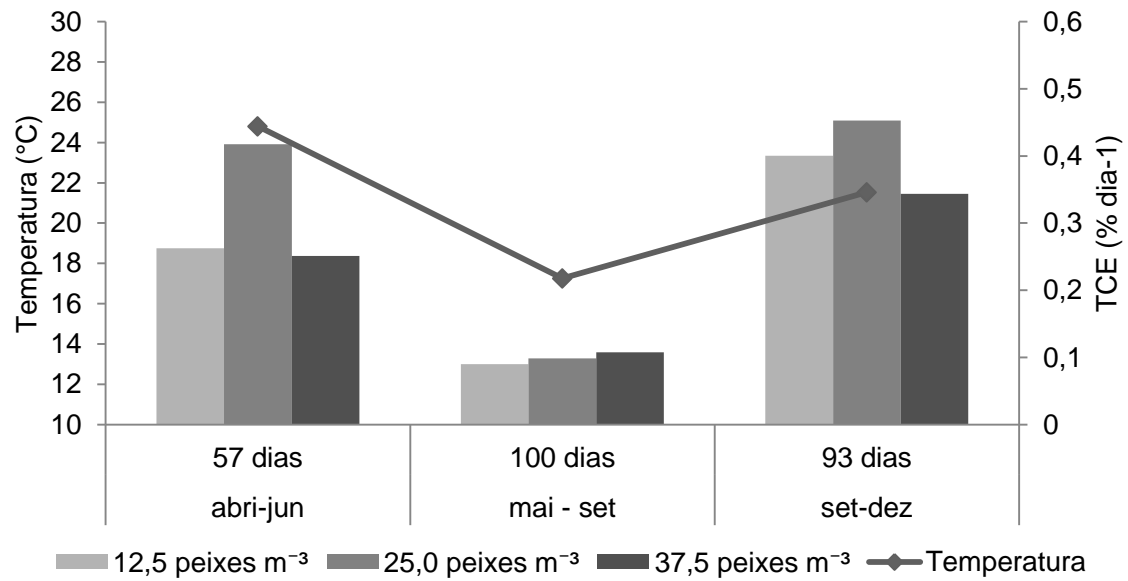
Figura 2. Variação da temperatura e da taxa de crescimento específico de Centropomus undecimalis entre biometrias intermediárias nas densidades 12,5, 25,0 e 37,5 peixes m -3 .
