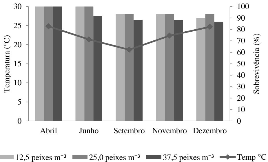
Figura 3. Variação da temperatura e da taxa de sobrevivência de robalo-peva ( Centropomus parallelus ) ao longo dos meses de cultivo nas densidades 12,5, 25,0 e 37,5 peixes m -3 .
